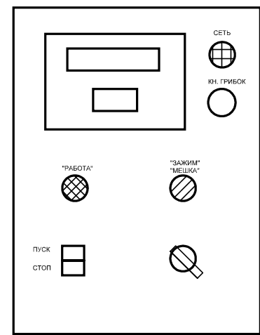
расположение элементов на передней панели шкафа
