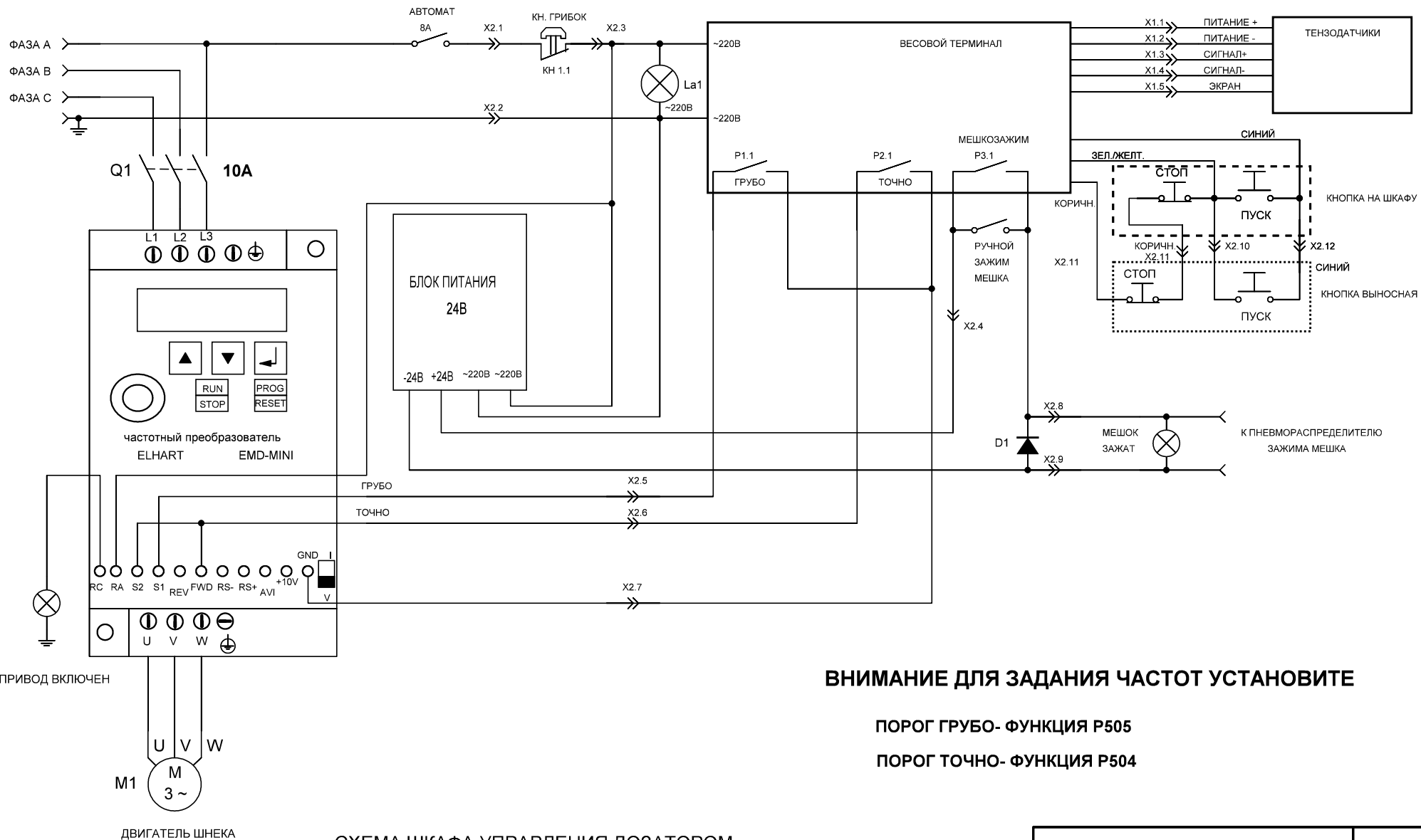
СХЕМА ШКАФА УПРАВЛЕНИЯ ДОЗАТОРОМ С ЧАСТОТНЫМ ПРИВОДОМ
